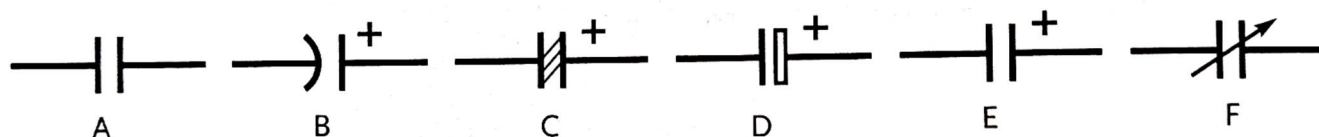
Rys. 2.46. Symbole kondensatorów: A – niespolaryzowany, B–E – spolaryzowane, F – zmienny (strojeniowy)
