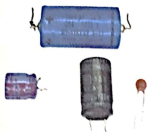
Rys. 2.47. Przykłady kondensatorów: a) elektrolitycznych i ceramicznego (po prawej, w formie pastylki), b) foliowych, c) tantalowych
